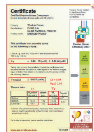
► Wyniki obliczeń stolarki okiennej w programie PHPP
