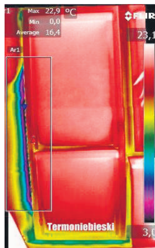
► Nieszczelność między ramą a skrzydłem okna
