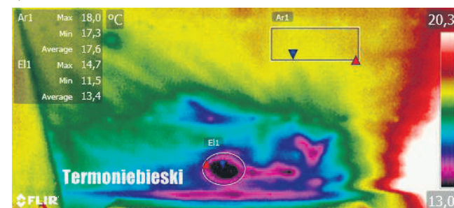
► Ubytek izolacji w sośnym dachu
